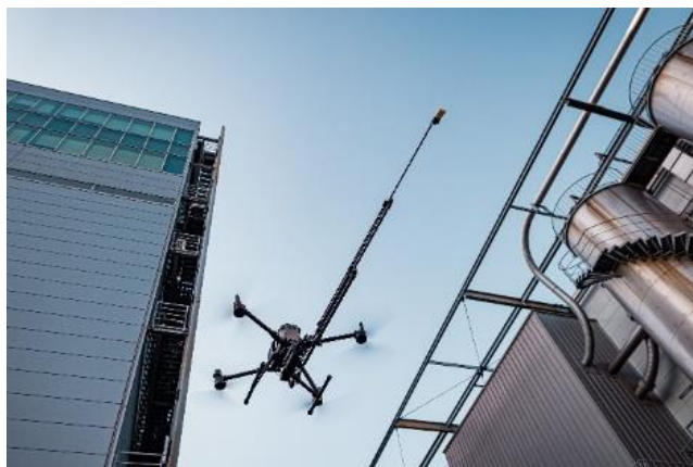
多目的伸縮装置「NYOI」
