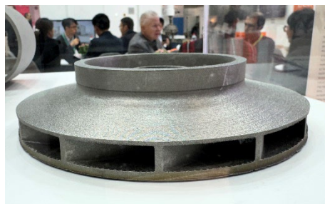
サポート材不要の造形事例 金属製ポンプ羽根車
