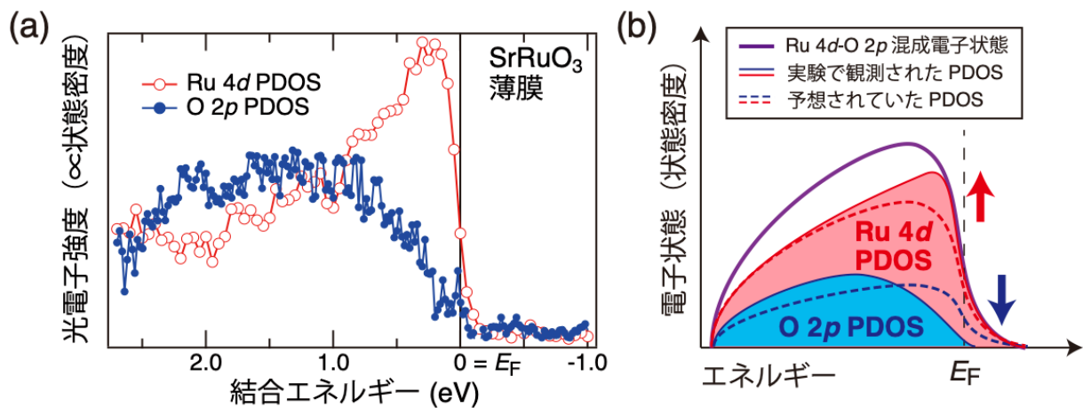
図 1：機能性酸化物 \text{SrRuO}_3 の電子状態
