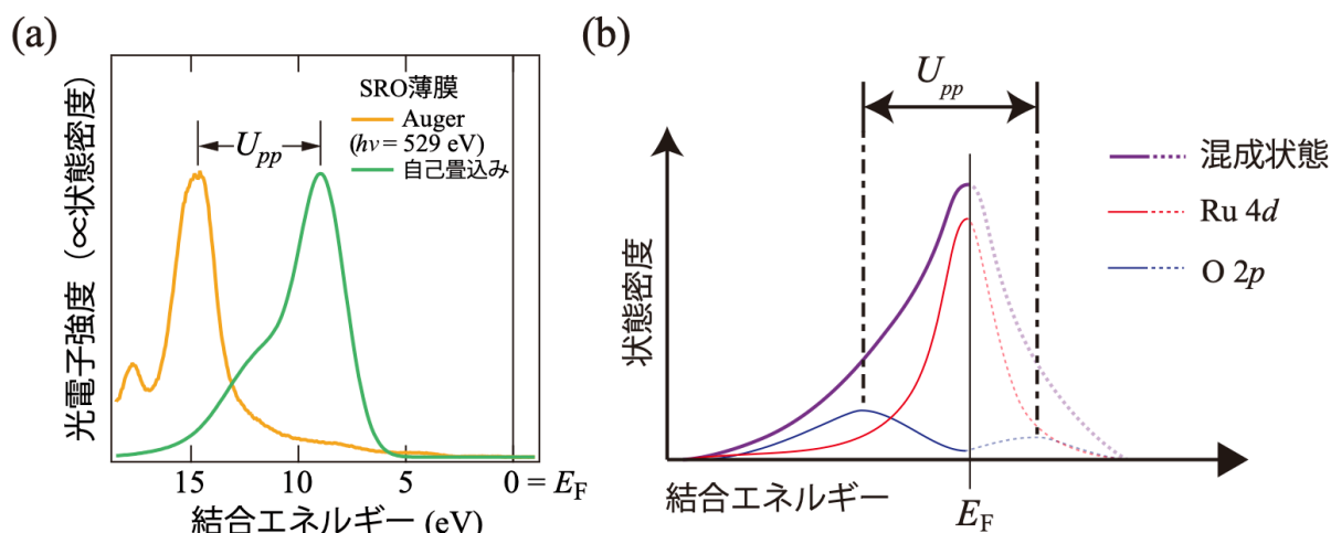
図 2 : SrRuO 3 における酸素の電子相関 ( U_{pp} )
