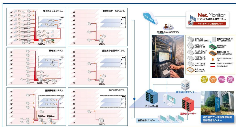
<ネットワーク構成イメージ図>
