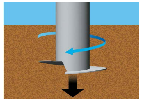
図1 回転による貫入施工
