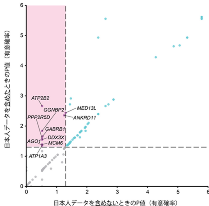
図：各遺伝子に認めた機能的 de novo 変異の数を統計的に検討して得られた P 値（この値が小さいほど、観察された機能的 de novo 変異の数が期待値よりも多いことを示す）をプロットした結果。日本人データを含めた場合、含めない場合の両方を検討し、縦軸に日本人データを含めたときの P 値（ -\log_{10} 変換したもの）、横軸に含めないときの P 値が示されている。破線は、統計学的に有意な水準（有意確率 5%；調べた遺伝子の数に伴う多重検定の問題を考慮した値）を示している。すなわち、ピンク色の背景で示した部分に含まれる、日本人データを含めないときには P 値が有意でないが、含めると有意になる 10 遺伝子（ ATP2B2 など）は、新規原因遺伝子候補といえる。
