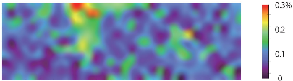
図2 図1の四角形部分の硫黄(a)、塩素(b)、亜鉛(c)の元素分布図。赤色の部分にこれらの元素の濃集が見られる。
