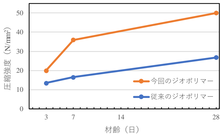
図2 ジオポリマーコンクリートの圧縮強度（大林組社内比較）
