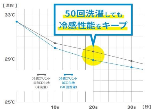
第三者機関による冷感プリントの洗濯耐久性能試験グラフ（10秒ごとの温度経過）
