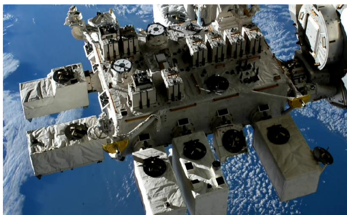
図2 ISS 船外曝露プラットフォーム (C)JAXA/NASA
