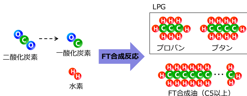
図1 FT合成反応
