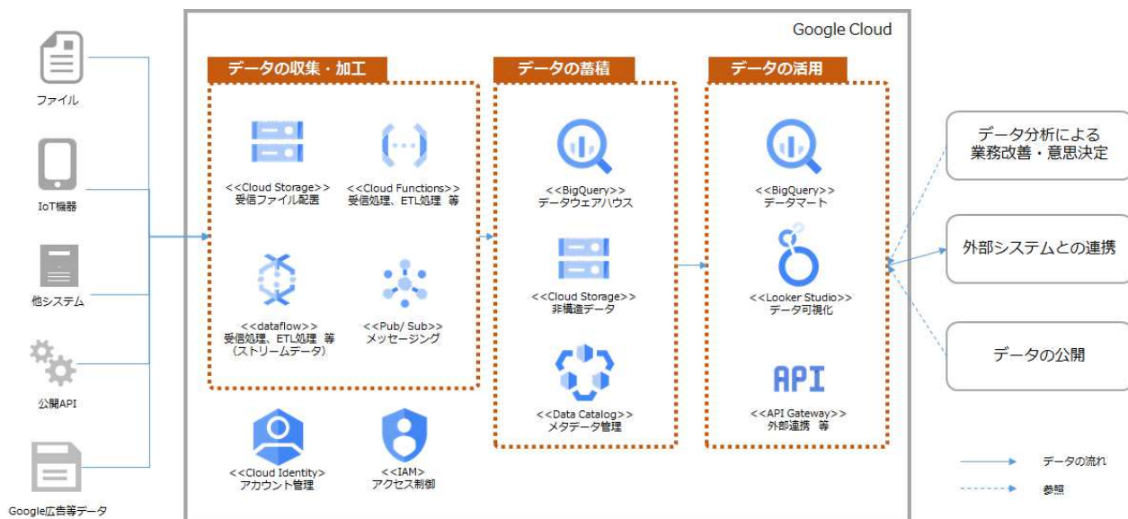
データ活用基盤構成図
