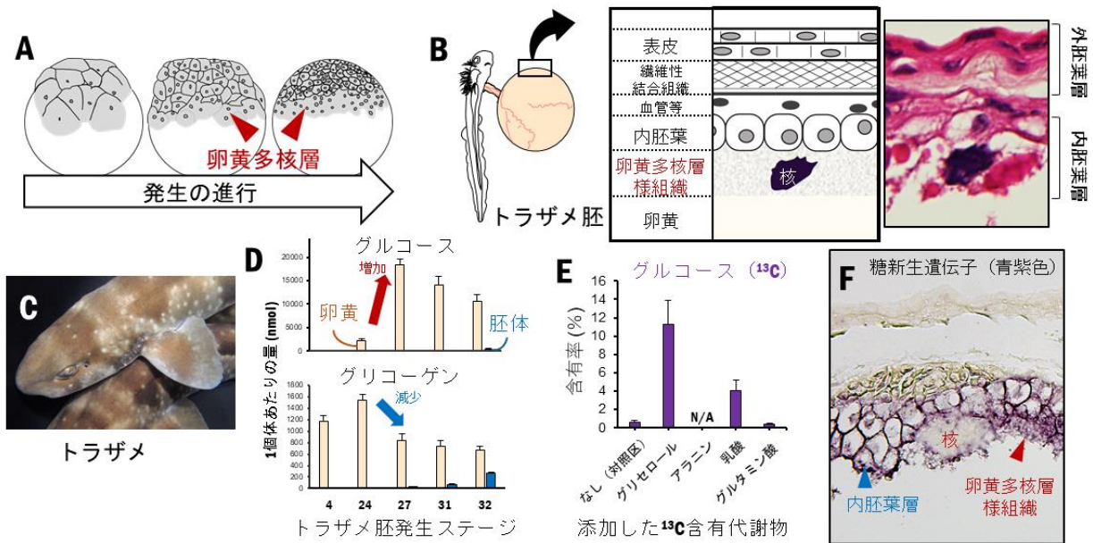
図 3. (A)ゼブラフィッシュやクサダマを含む真骨魚類で卵黄多核層が形成される過程。一部の細胞が卵黄表面の細胞質と融合して卵黄多核層を形成する。(B)トラザメ卵黄囊の表面付近の断面図。卵黄多核層様組織を含むさまざまな組織が存在する。(C)トラザメ成魚（写真提供：下山紘也 東京大学大気海洋研究所・博士課程）。(D)発生過程の卵黄囊でグルコースが増加していた。グリコーゲンはわずかに減少するものの、その量はグルコースと比較して非常に少なかった。(E)卵黄囊表面付近の組織を用いた培養実験。 ^{13}C で構成されたグリセロールを培養液に添加したときに最もグルコース ( ^{13}C ) が検出された。N/A：データ採取不可能。(F)糖新生に関する遺伝子の発現。発生後期では、卵黄多核層様組織と内胚葉層で発現が確認された。
