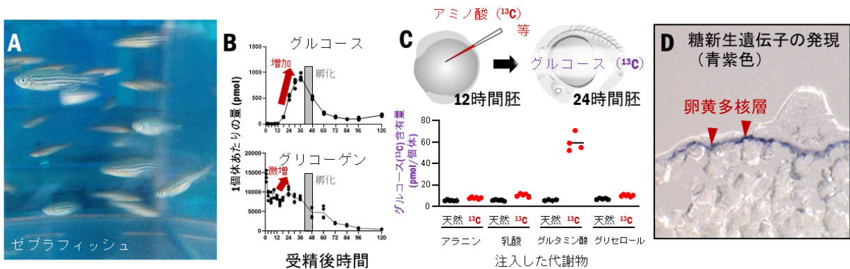
図 1. (A)ゼブラフィッシュの成魚。(B)受精後12時間以降、グルコースとグリコーゲンが同時に増加していた。(C) (上段) 炭素 13 ( ^{13}\text{C} ) で構成された代謝物を卵黄に注入し、これの一部がグルコースに変化するかどうかを調べる実験を行った。(下段) グルタミン酸 ( ^{13}\text{C} ) を注入したときに最もグルコース ( ^{13}\text{C} ) が検出された。天然の各代謝物を比較対象として使用した。(D)糖新生に関連する遺伝子の発現。卵黄多核層に遺伝子発現が検出された。
