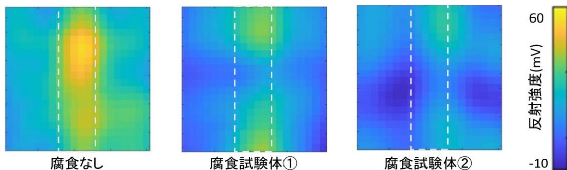
図1 腐食度評価
