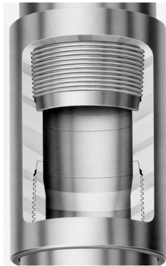
図 VAM®継手 概略図
